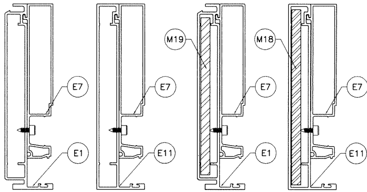
JAMB 'J1'
